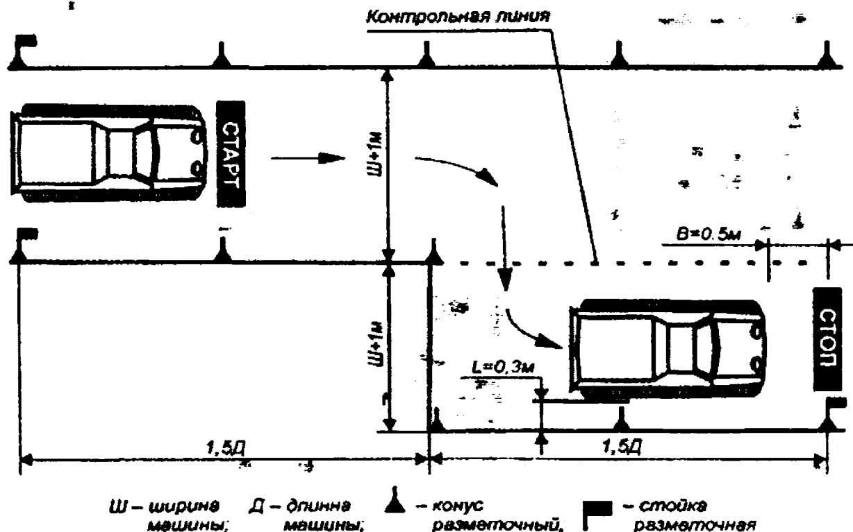
Рис. 8. Остановка для безопасной посадки или высадки пассажиров, загрузки-выгрузки СМ технологическими материалами
