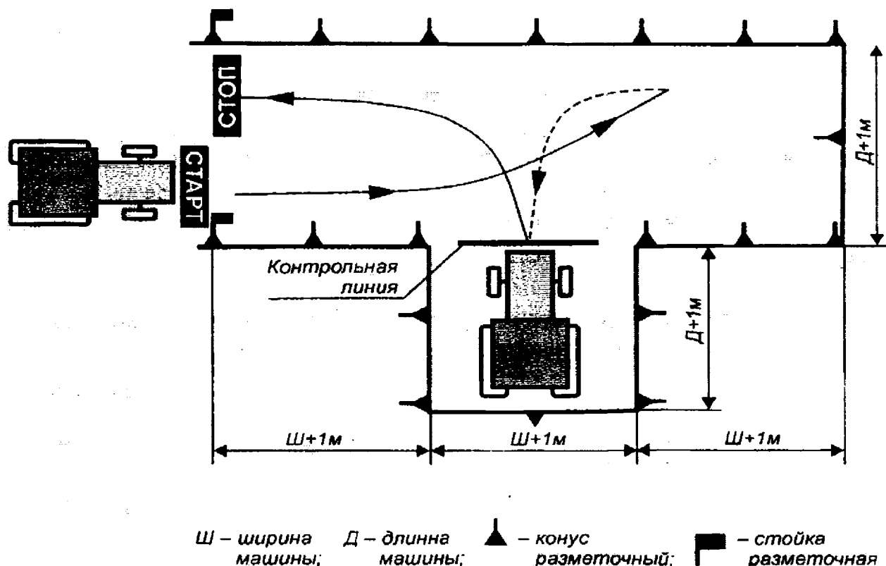
Рис. 9. Постановка самоходной машины в «бокс» задним ходом
