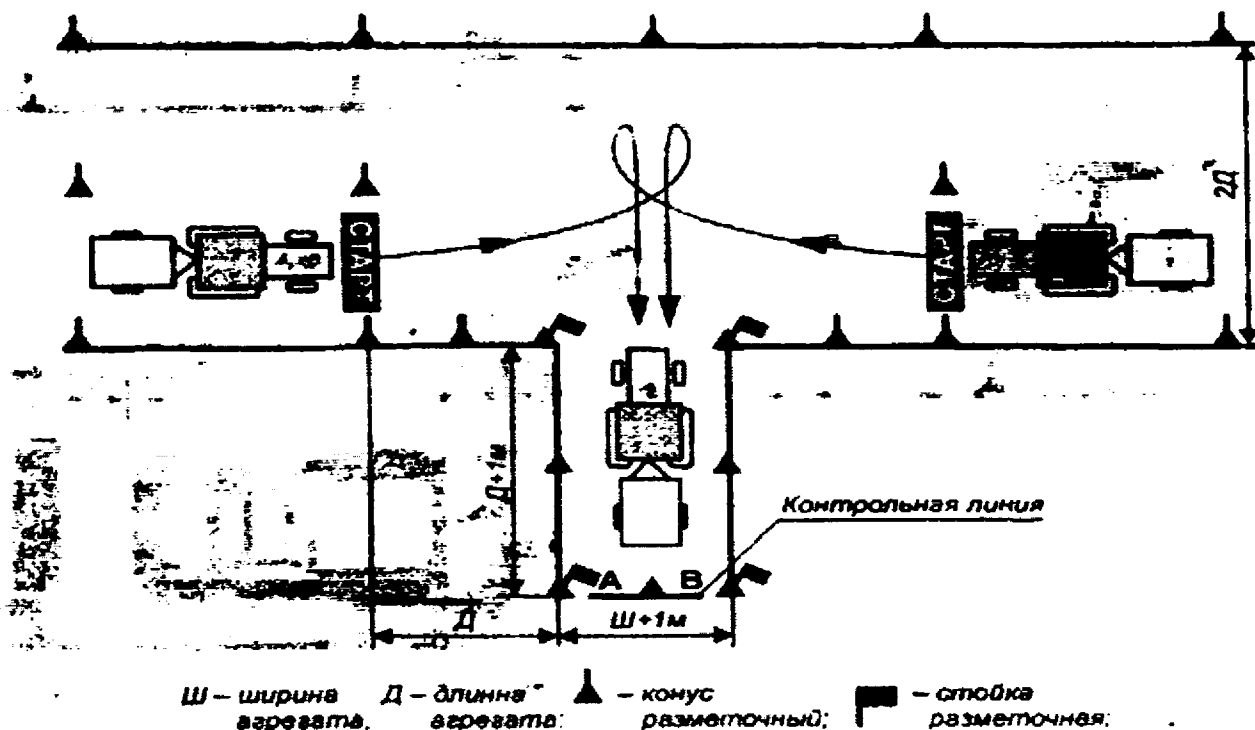
Рис. 7. Движение задним ходом, въезд в "бокс" в агрегате с прицепом
