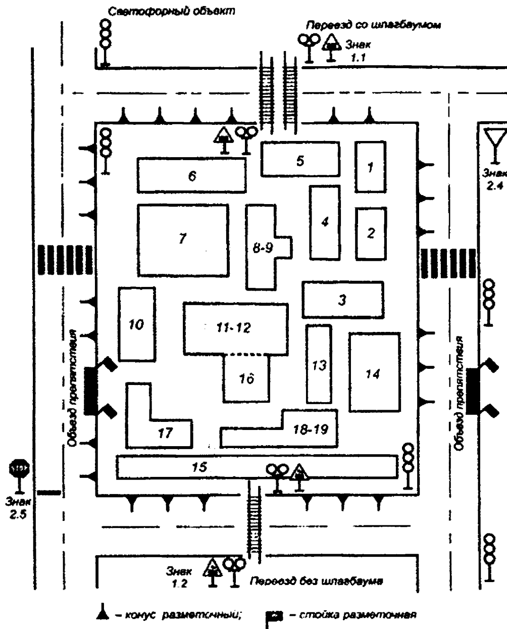
Рис. 1. Схема площадки для проведения практического экзамена
