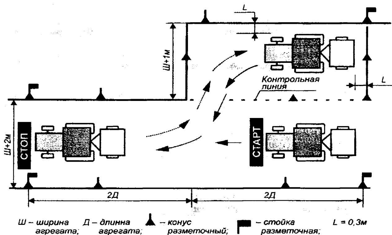
Рис. 19. Парковка СМ с прицепом задним ходом и выезд с парковочного места, параллельная парковка
