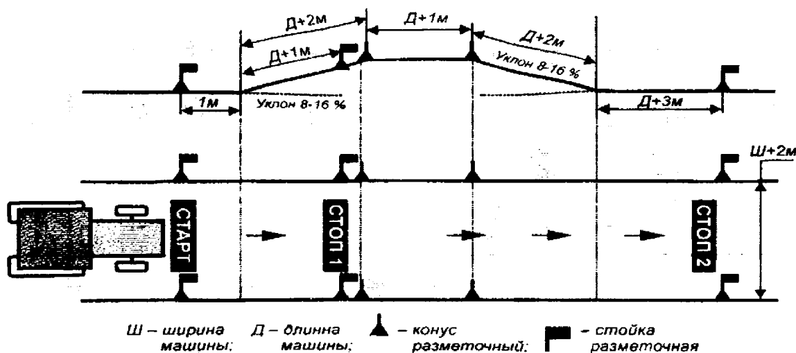
Рис. 4. Остановка и трогание на подъеме
