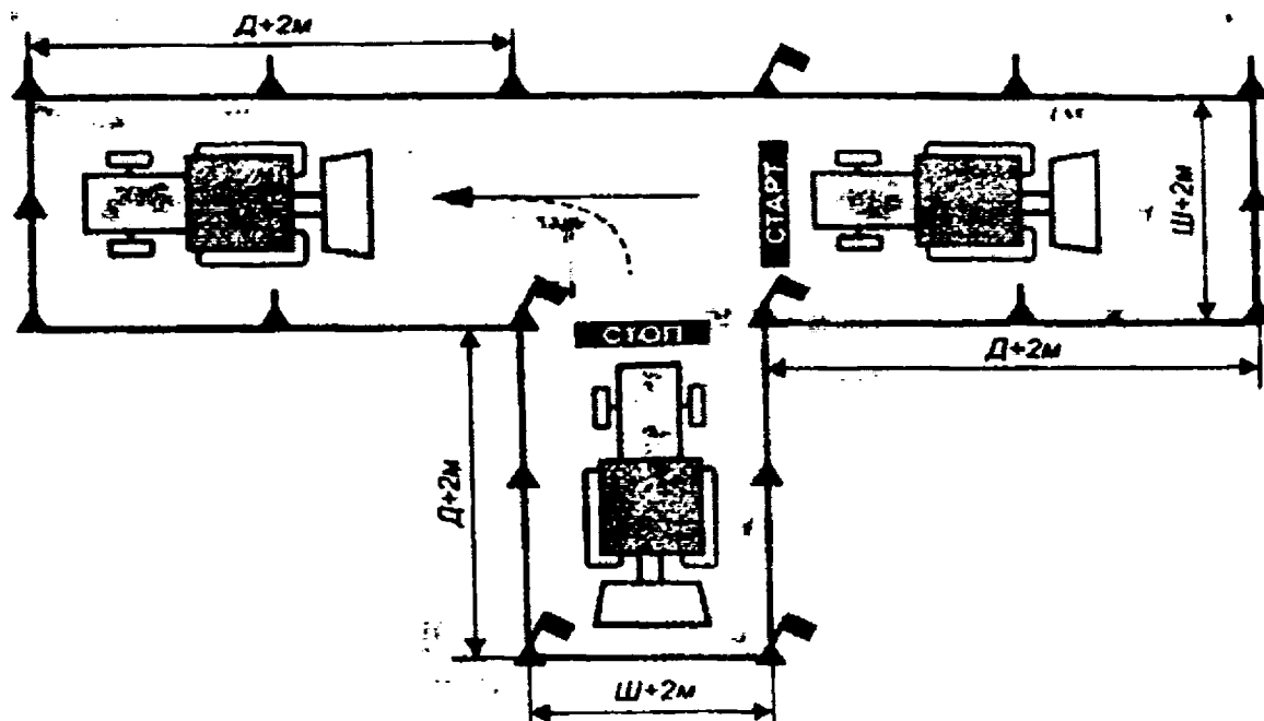
Рис. 9. Агрегатирование с навесной машиной или прицепом
