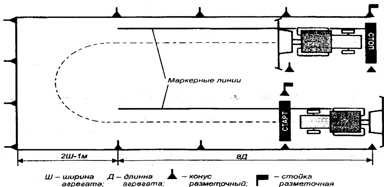
Рис. 15. Движение по маркерной или «провешенной» линии
