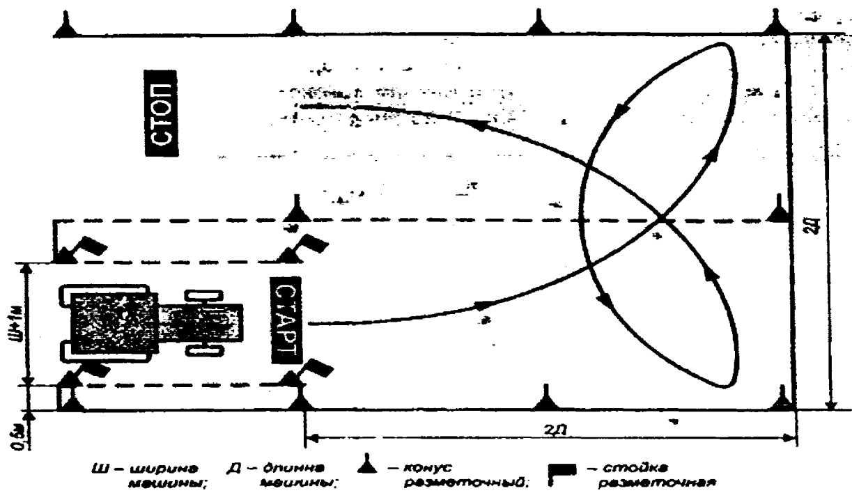
Рис. 5. Разворот маневрирование в ограниченном пространстве
