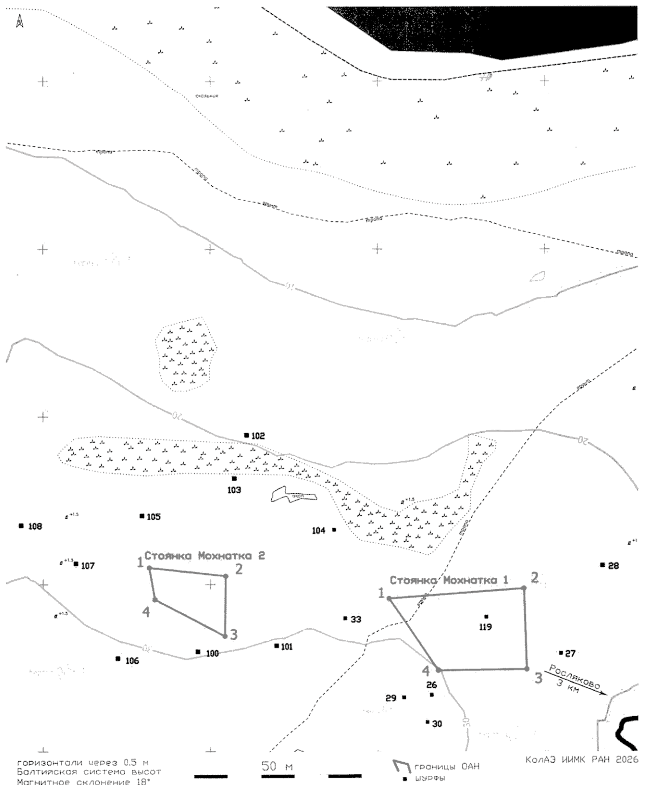
Топографическая съемка. Масштаб 1:1000
